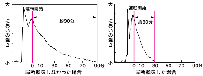
局所排気の有無によるにおいの減衰効果
