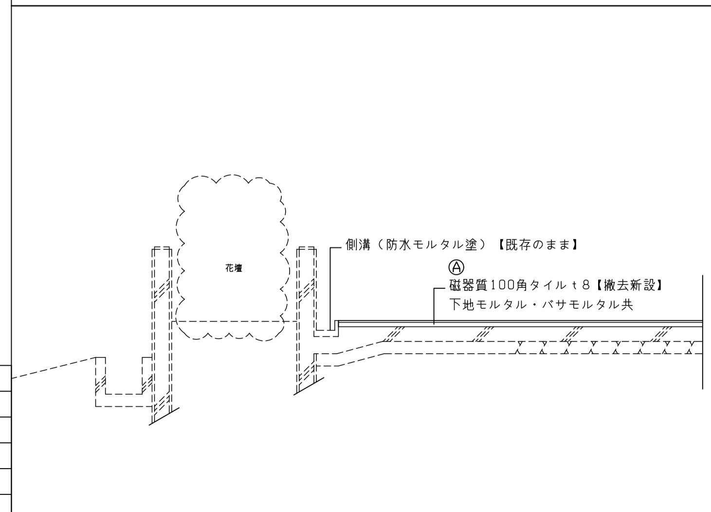
a断面詳細図
