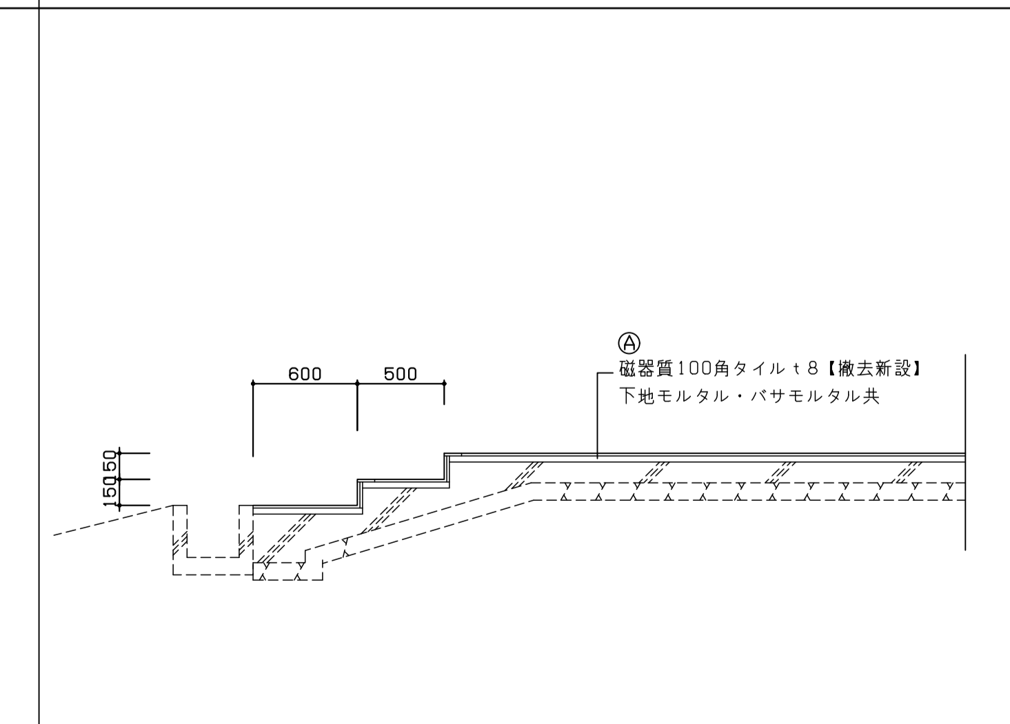
b断面詳細図
