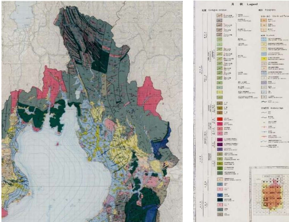
図 長浜市の地質図
