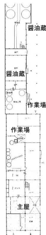
白木屋醤油店 平面図
