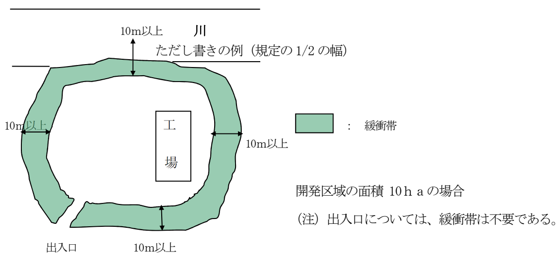
図 7-1 緩衝帯配置図 (案)
