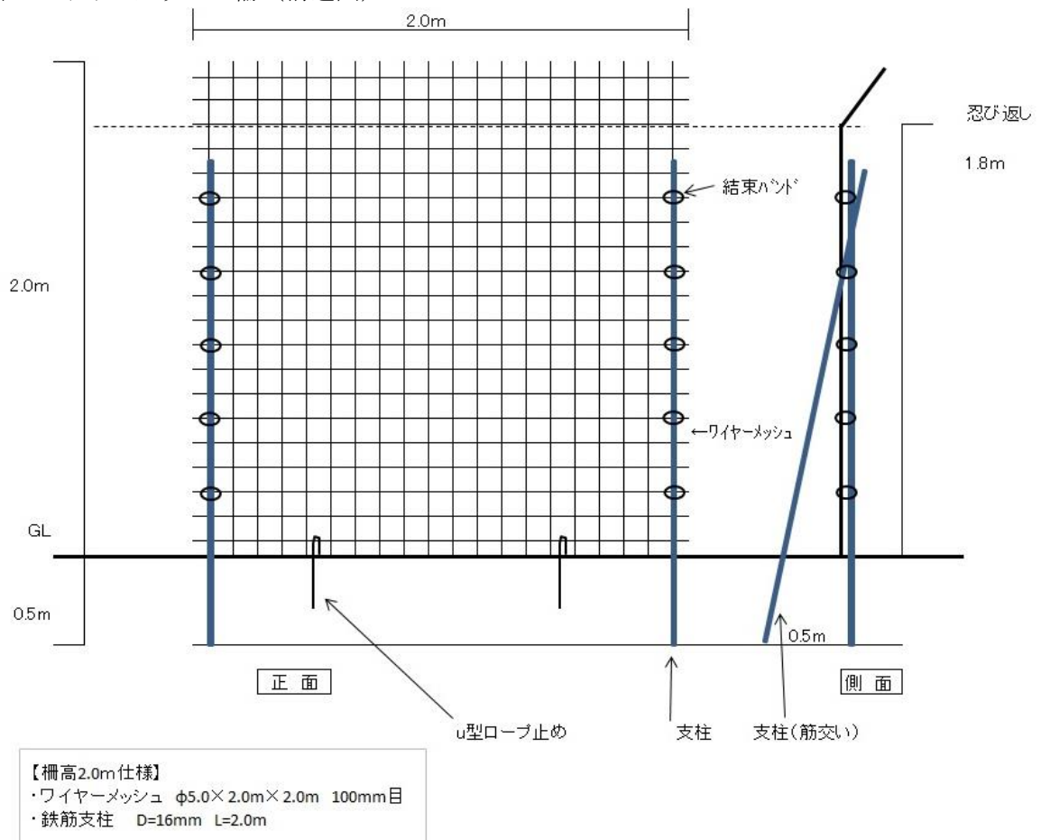
別図 ワイヤメッシュ柵 (構造図)
