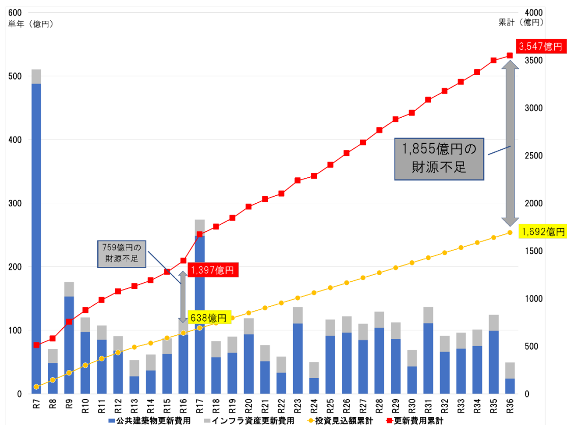
図33 公共施設等の更新費用推計グラフ
