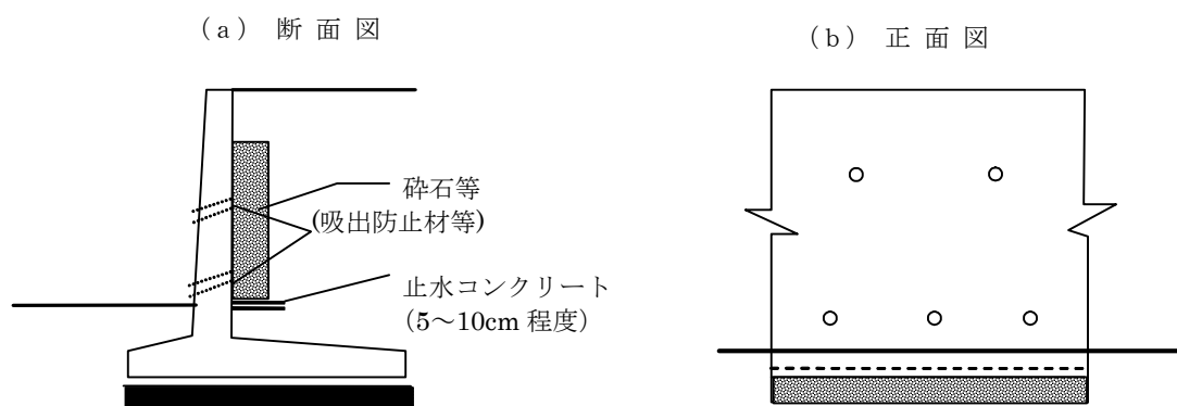
図11-21 水抜き穴の配置
