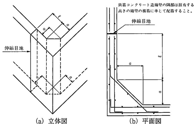
図11-18 隅角部の補強方法および伸縮継目の位置
