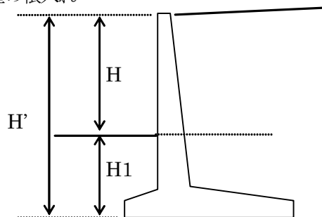
図11-23 擁壁の根入れ
