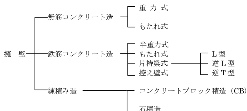
図11-9 擁壁の種類
