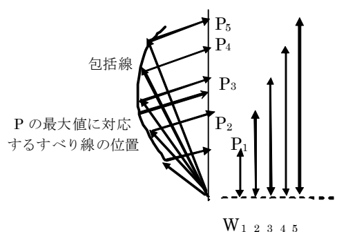
(d) 連力図の重ね合わせ
