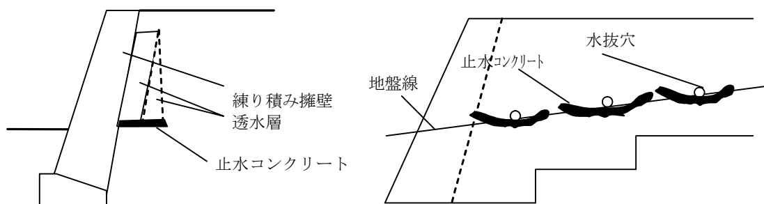
図11-22 止水コンクリート
