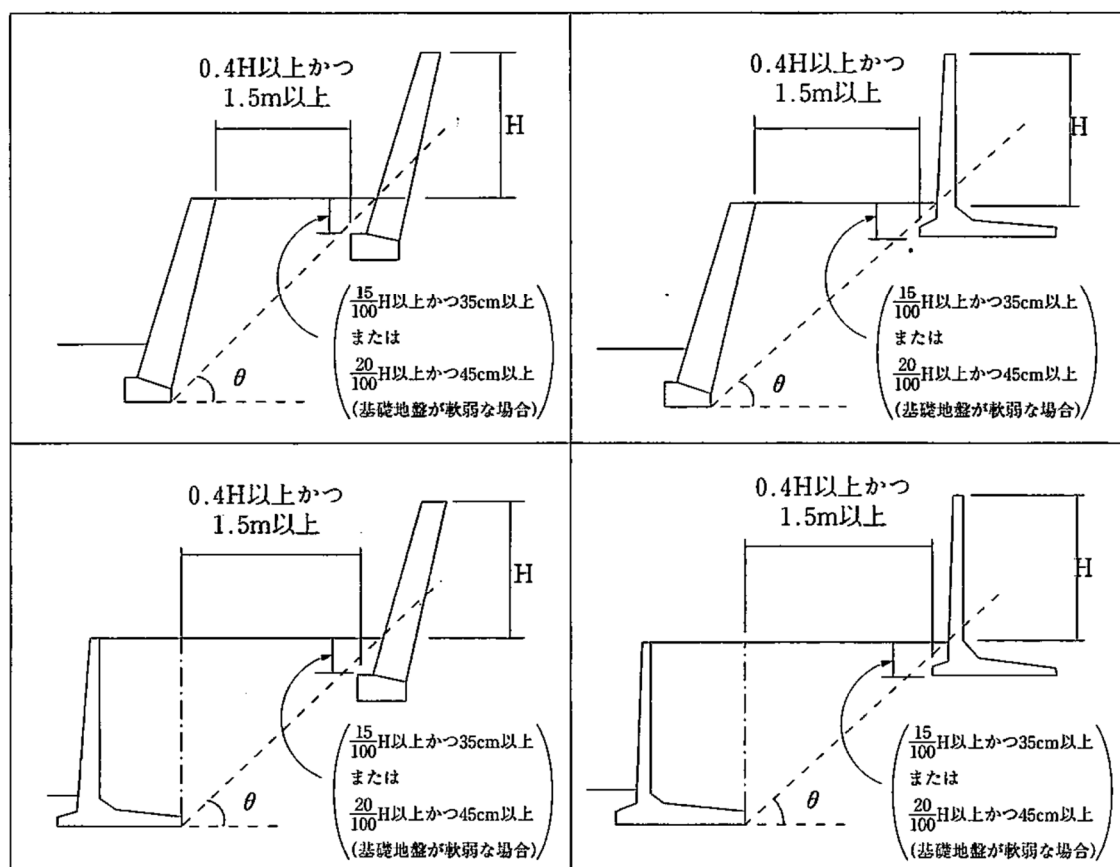
図11-8 上部・下部擁壁を接近して設置する場合
