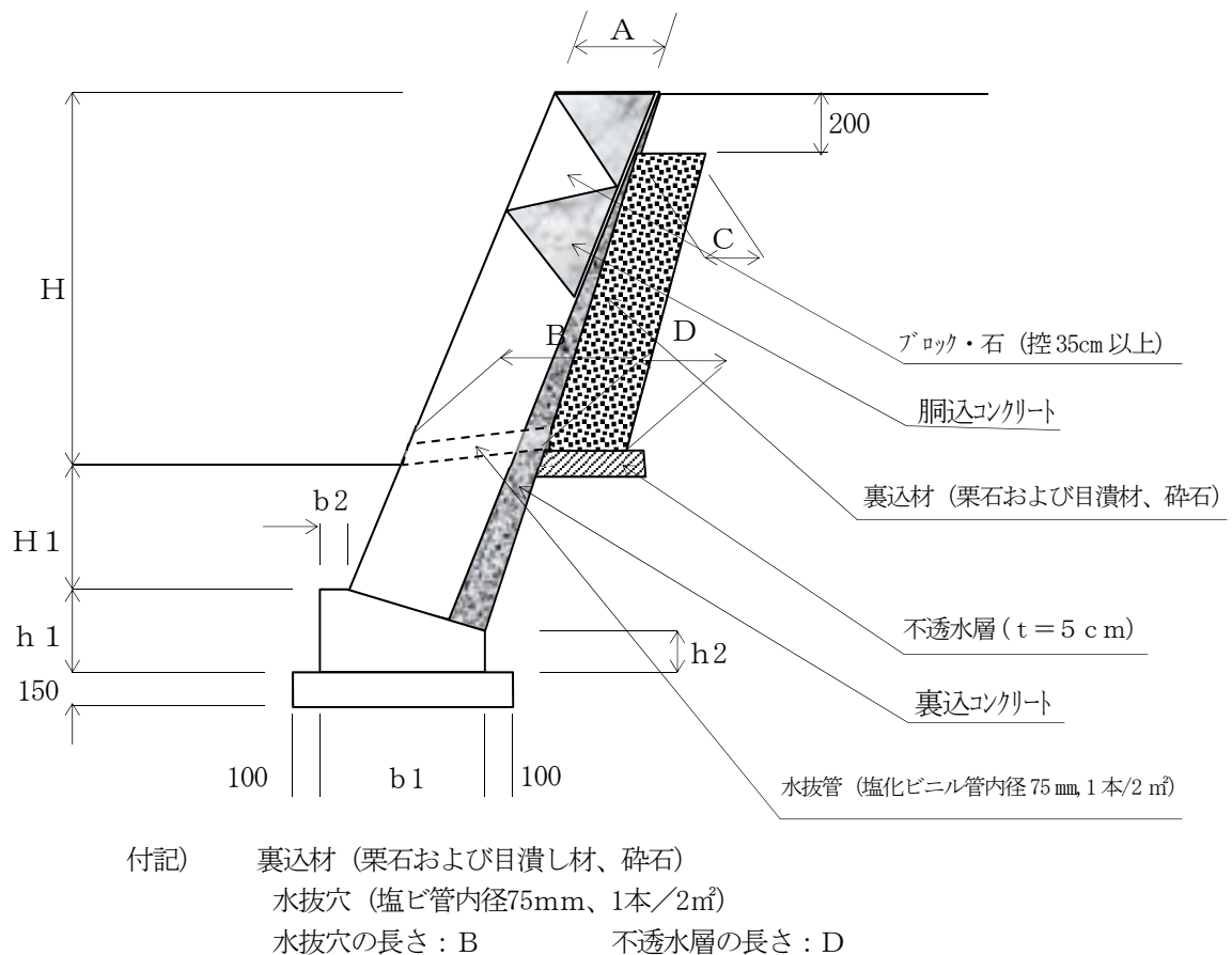
図11-14 練積み造擁壁の構造
