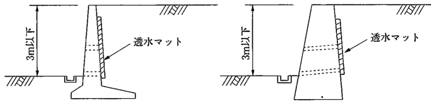
(a)擁壁の高さが3 m以下の場合
