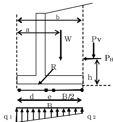
図11-13 地盤反力度の求め方
