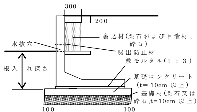
図11-20 プレキャスト擁壁標準断面図
