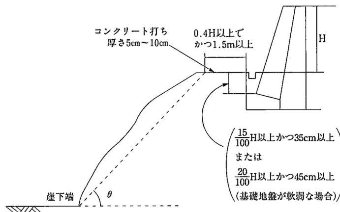
図11－7 斜面上に擁壁を設置する場合
