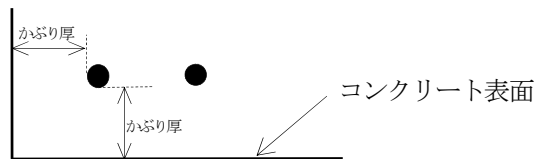
図11 - 19 鉄筋のかぶり
