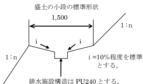
図11-6 盛土の小段
