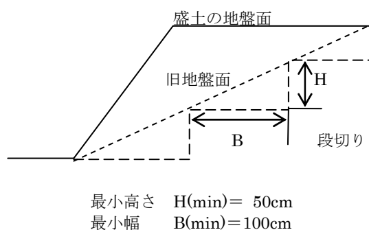
図11-3 段切り
