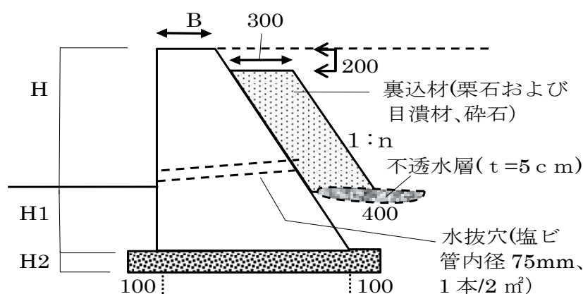
図11-17 重力式擁壁標準断面図
