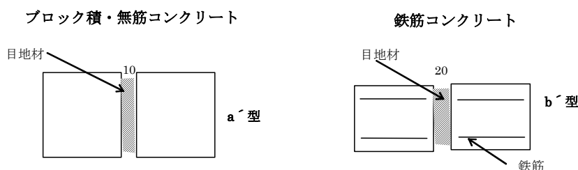
図11-26 伸縮目地
