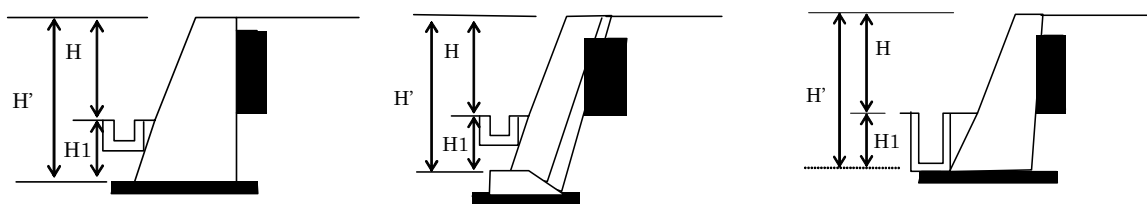
図11-24 排水構造物がある場合の根入れ
