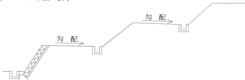
図 11-1 がけ面の排水
