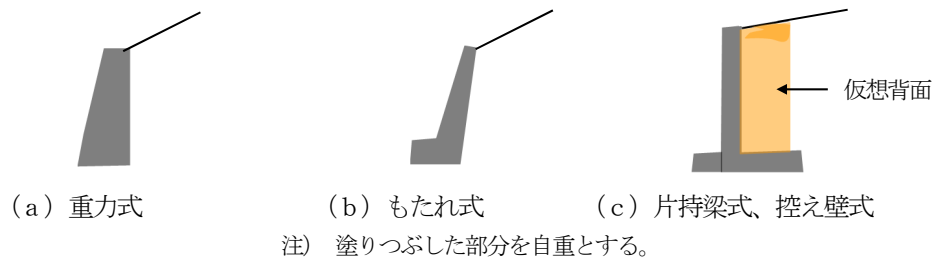
図11-10 擁壁の自重
