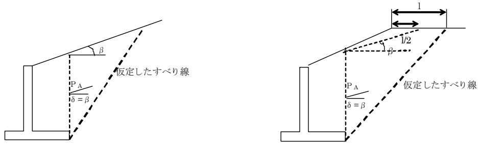
図11-12 \beta の設定方法
