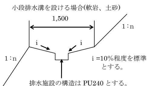
図11-6 盛土の小段
