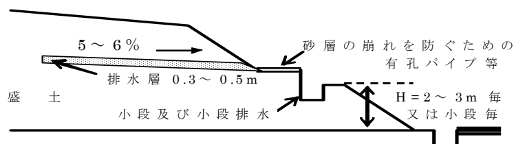
図11-4 水平排水層 (例)
