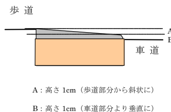
図3-12 歩道縁石
