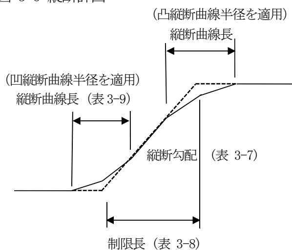
図 3-6 縦断計画
