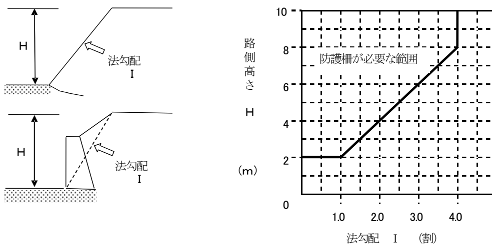
図 3-15 法勾配と路側高さの関係
