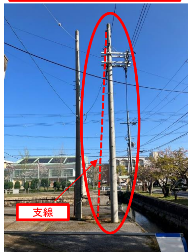
電柱3
