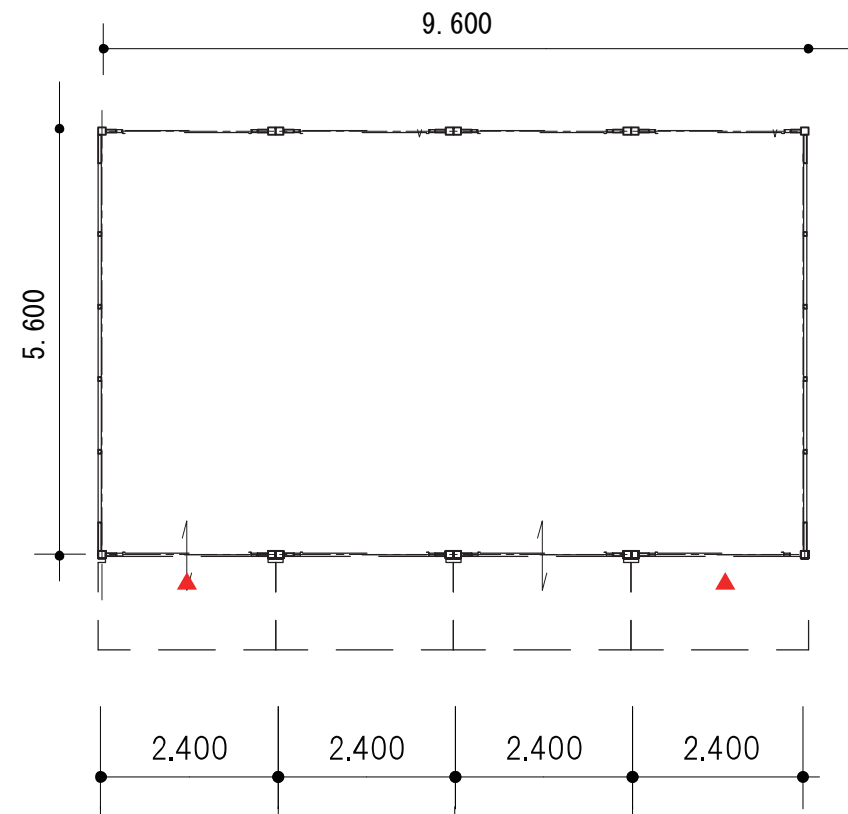
1階平面図
