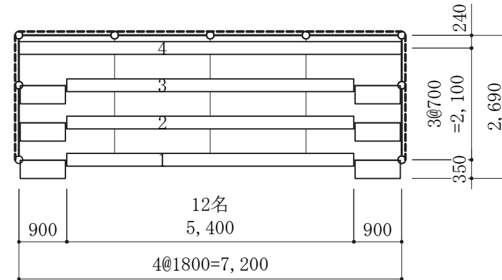
平面図 S=1/100 収容人員：48名×4基＝192名（座席当たり45cm／名試算）
