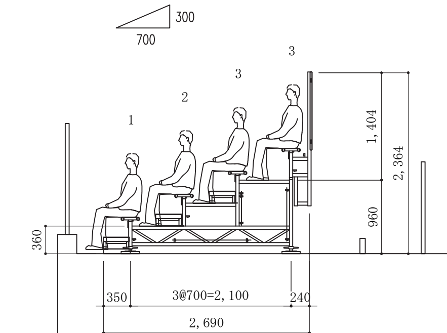
断面図 S=1/50
