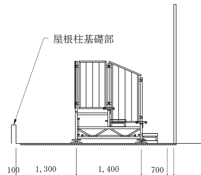
側面図 S=1/50
