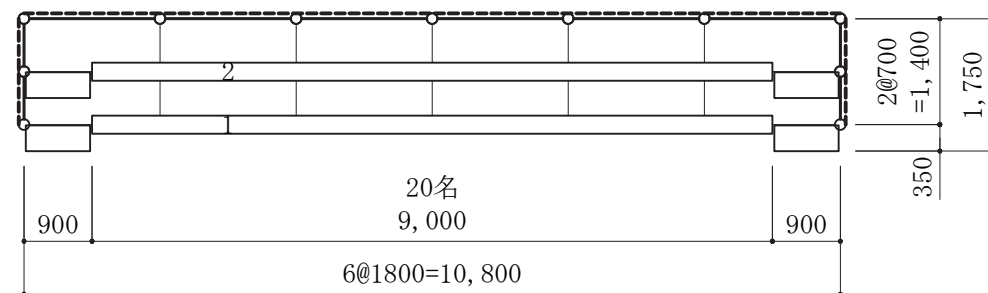
平面図 S=1/100 収容人員：40名×6基＝240名（座席当たり45cm/名試算）
