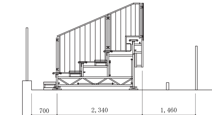
側面図 S=1/50
