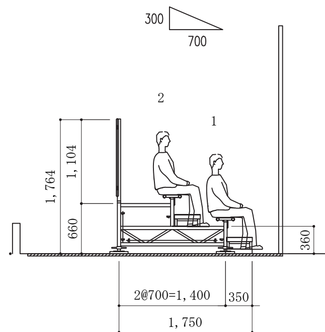
断面図 S=1/50
