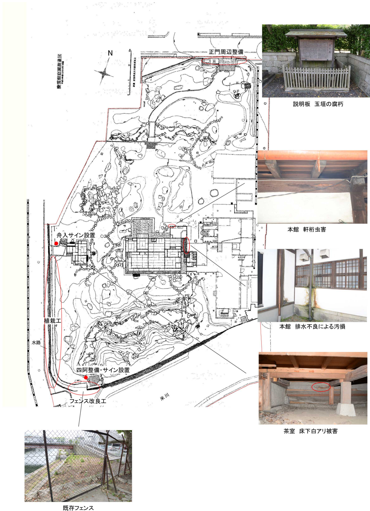
慶雲館 令和7年度保存整備位置図
