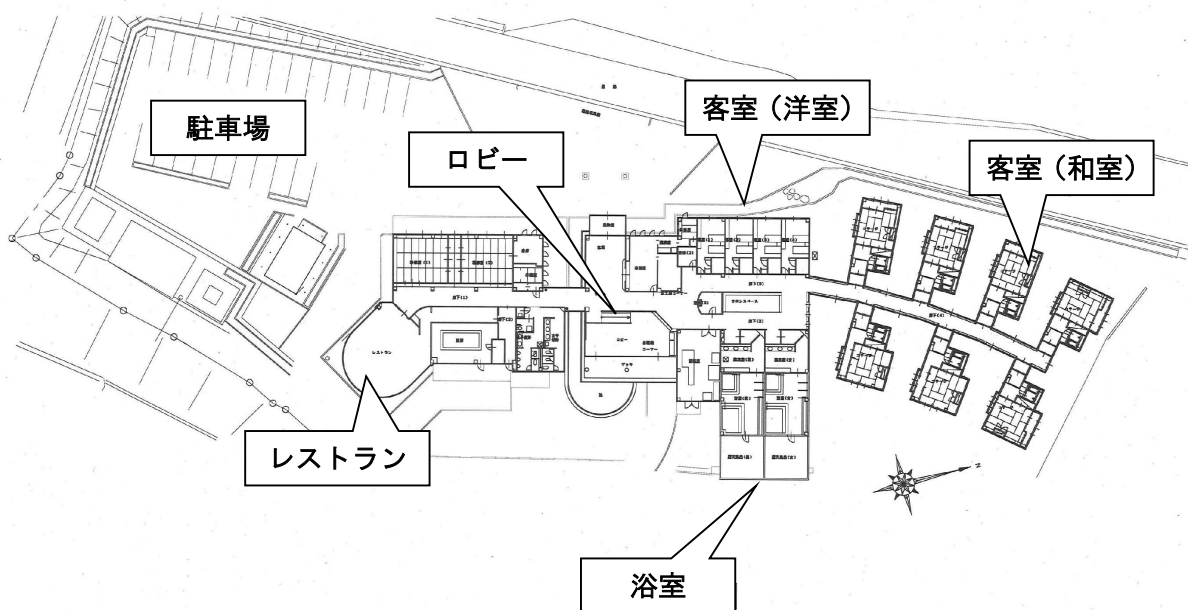
施設平面図
