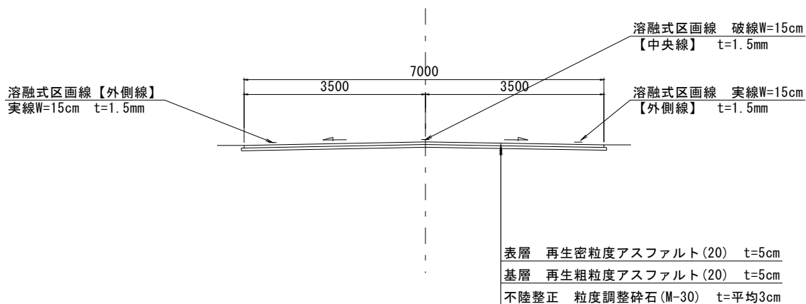
標準施工断面図
