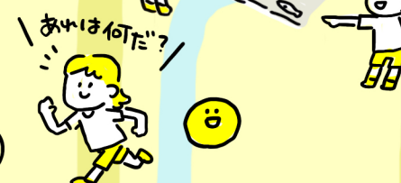
曳山博物館
