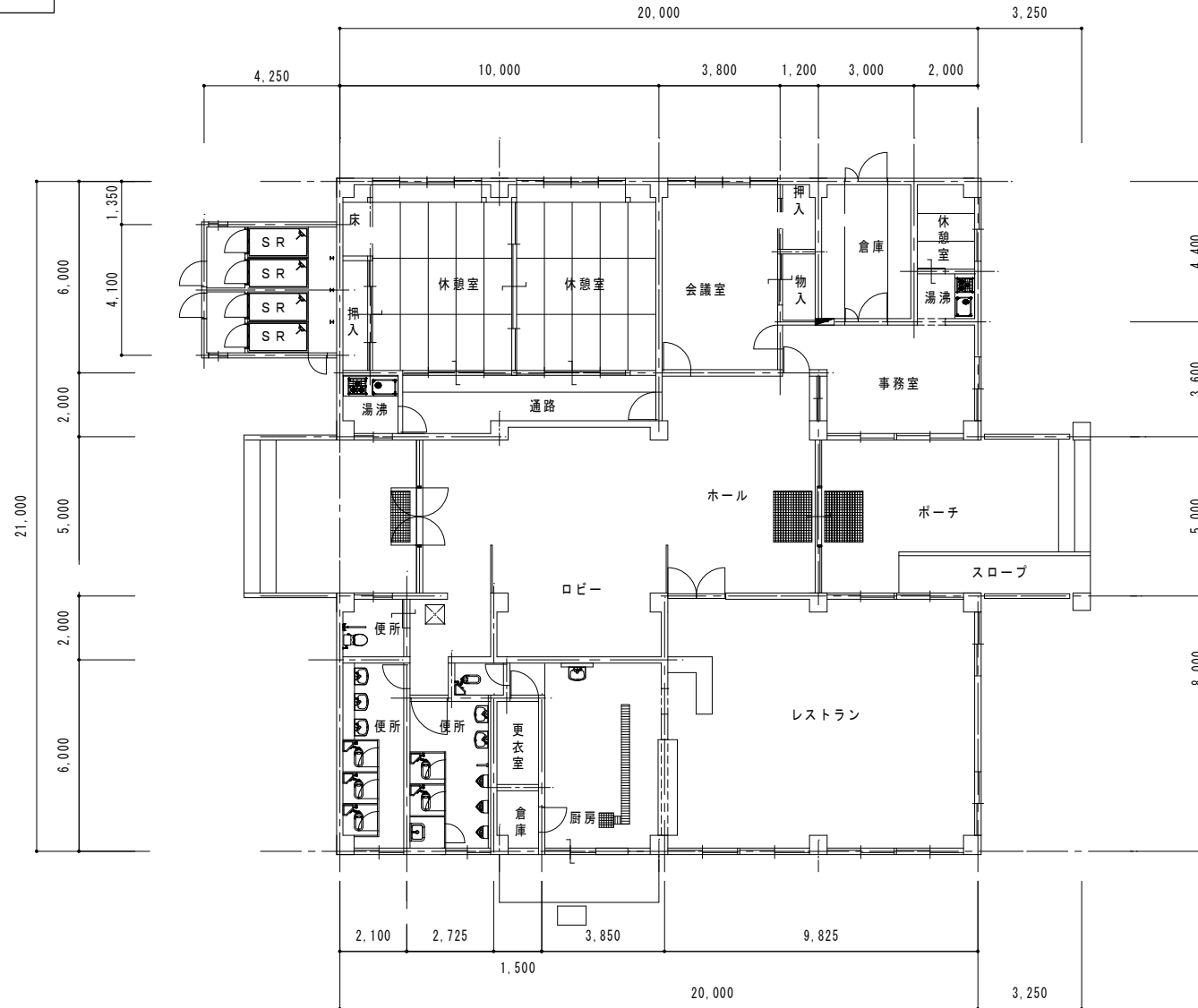
平面図 1/150
