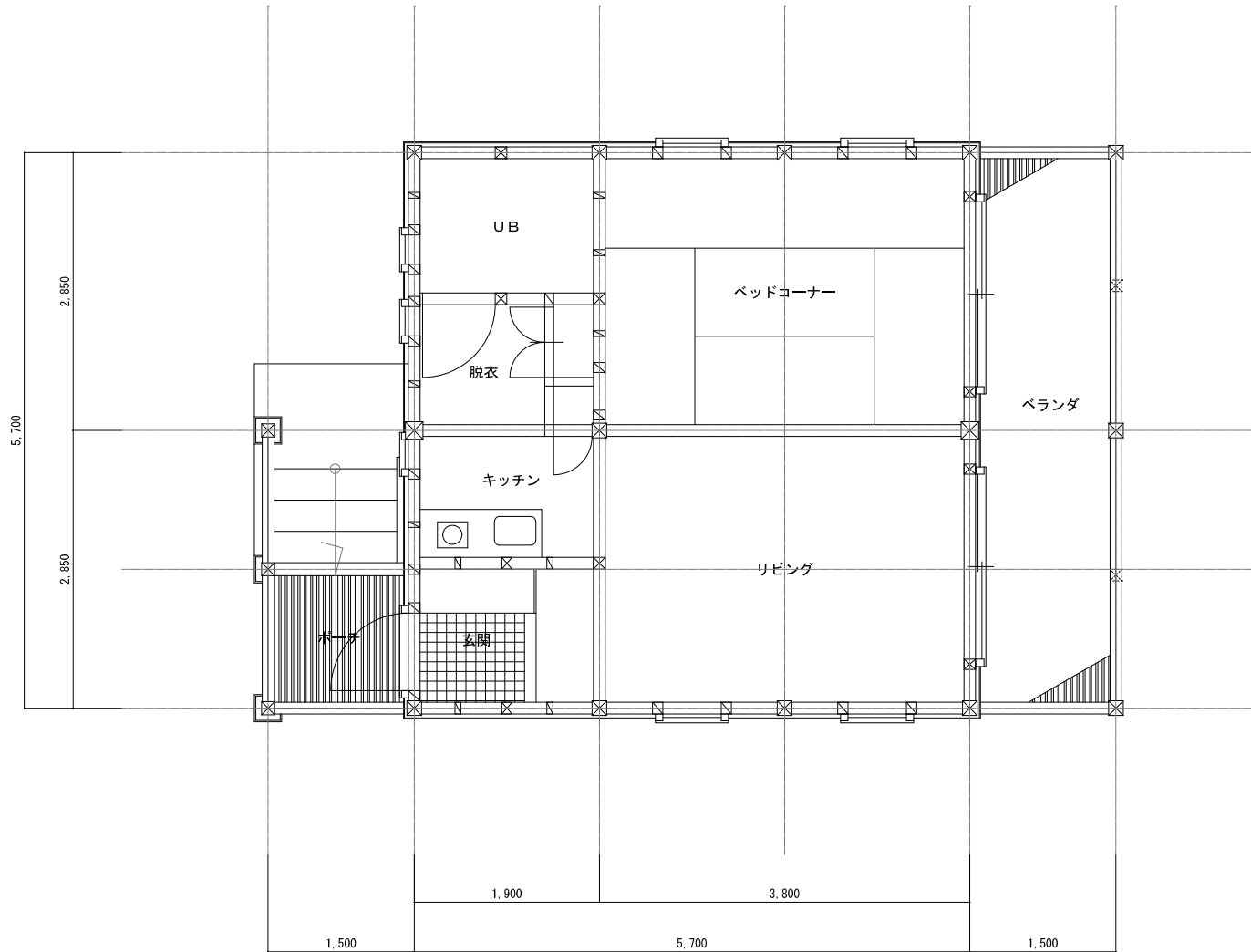
ヴィラA-2 1:50
