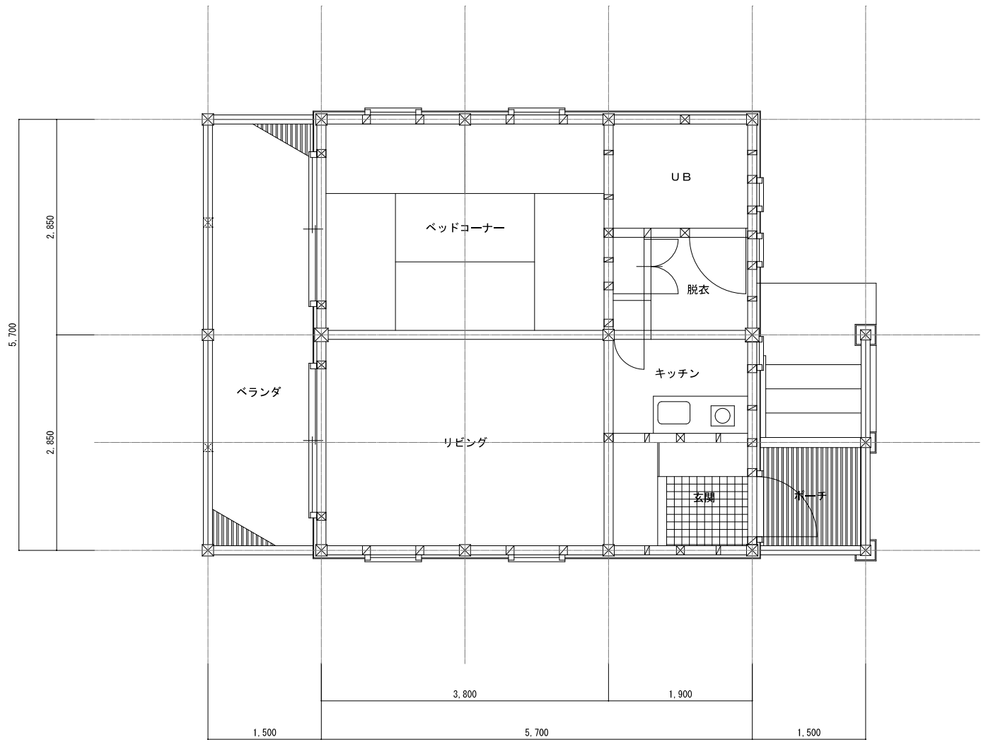
ヴィラA-1 1:50
