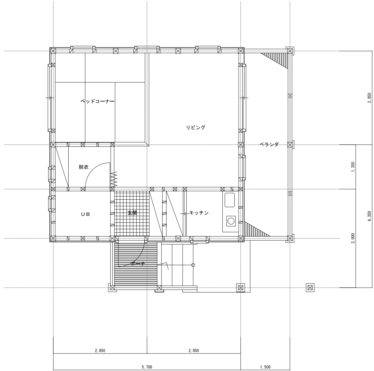
ヴィラB-1 1:50
