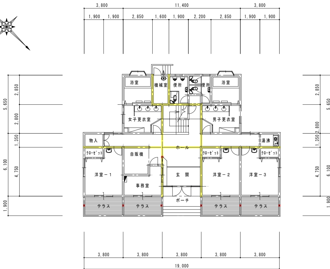
1 階 平 面 図 1/150
