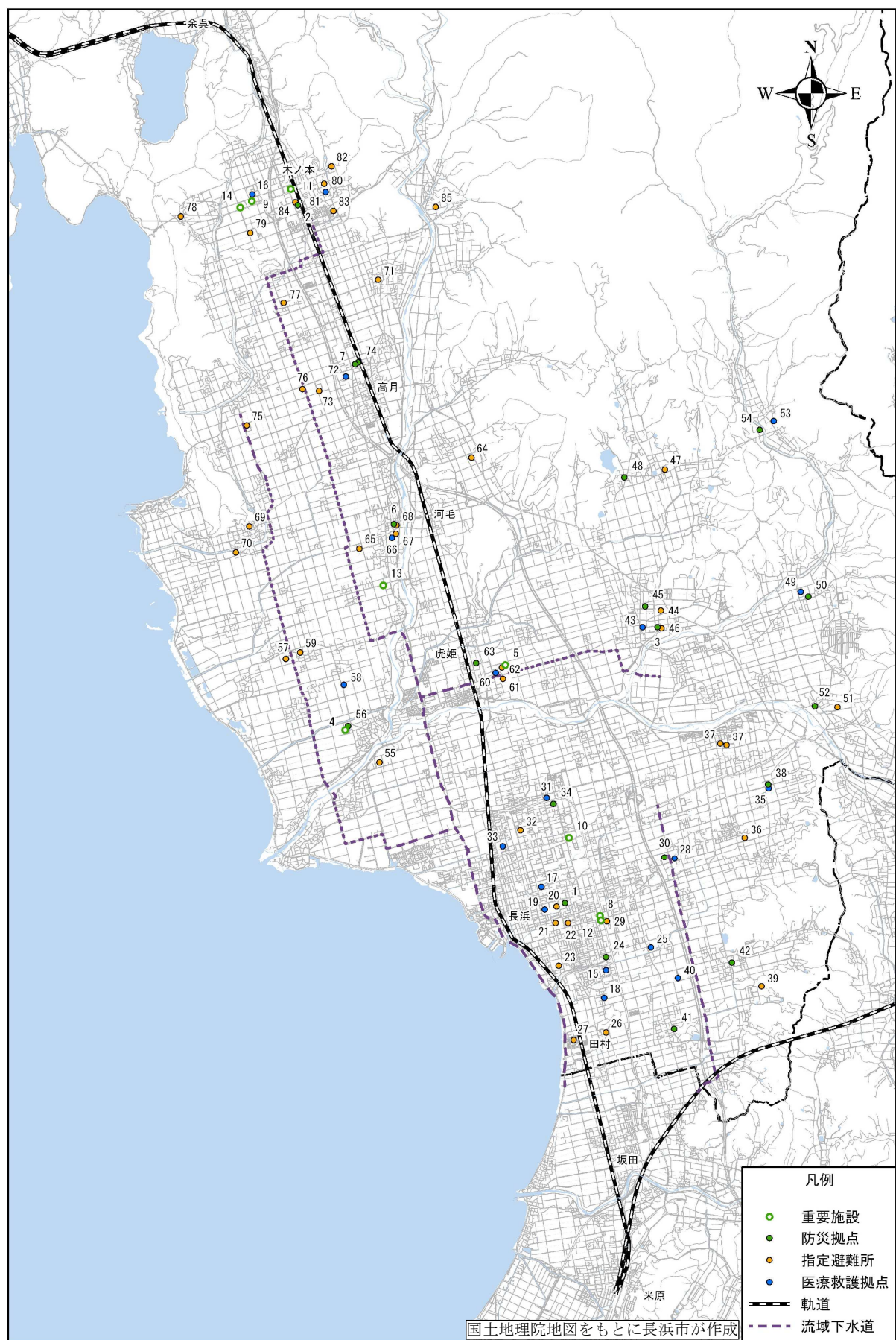
図 3.7 重要施設位置図
