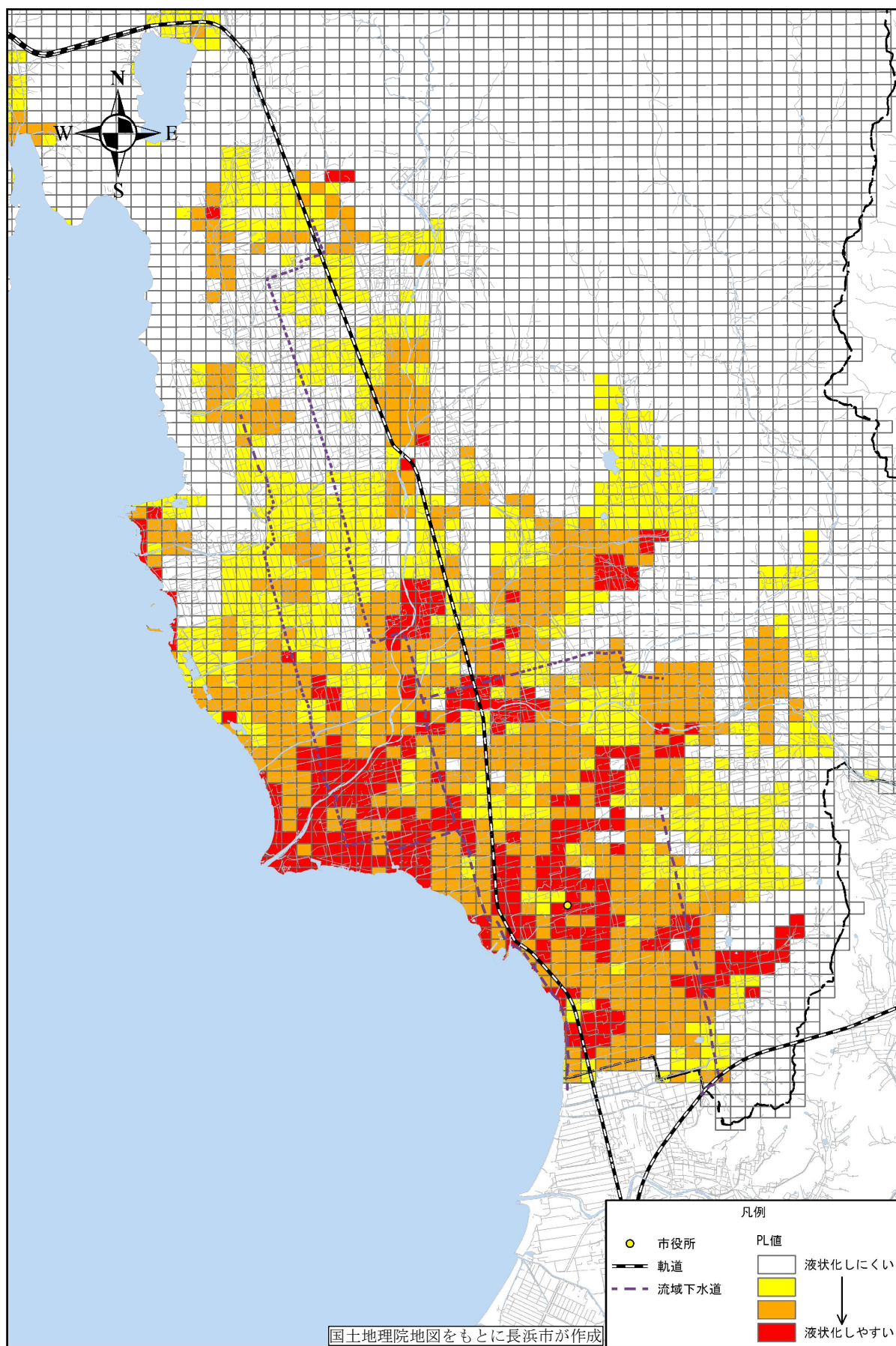
図 3.4 液状化のしやすさ分布図（南海トラフ地震）
