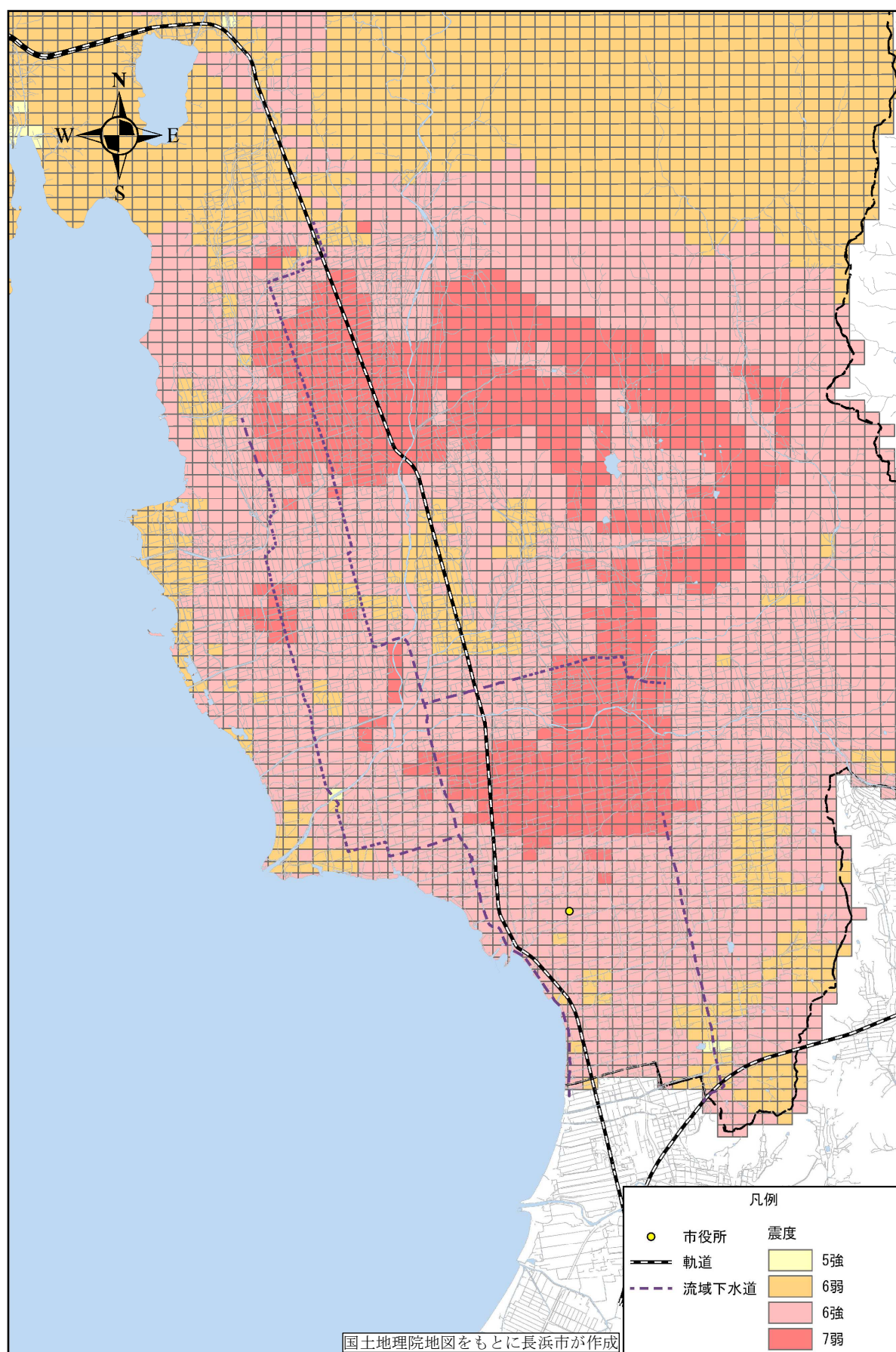
図 3.5 震度分布図（直下型地震：柳ヶ瀬・関ヶ原断層帯地震）
