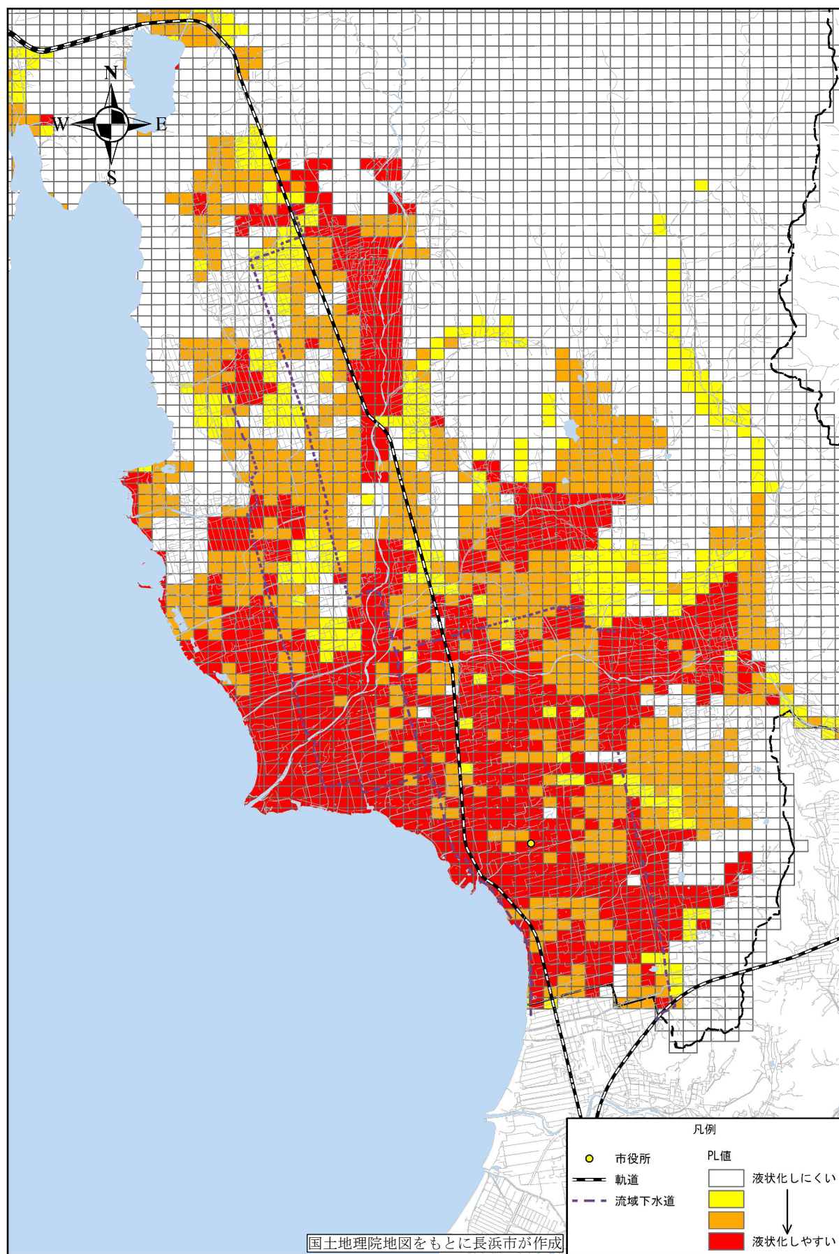
図 3.6 液状化のしやすさ分布図（直下型地震：柳ヶ瀬・関ヶ原断層帯地震）
